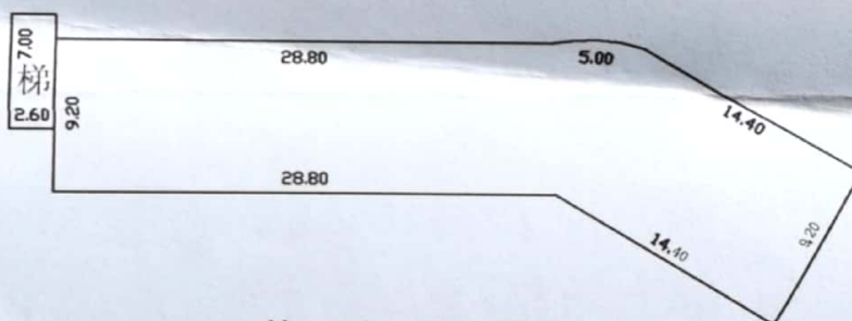
第一至二层平面图
