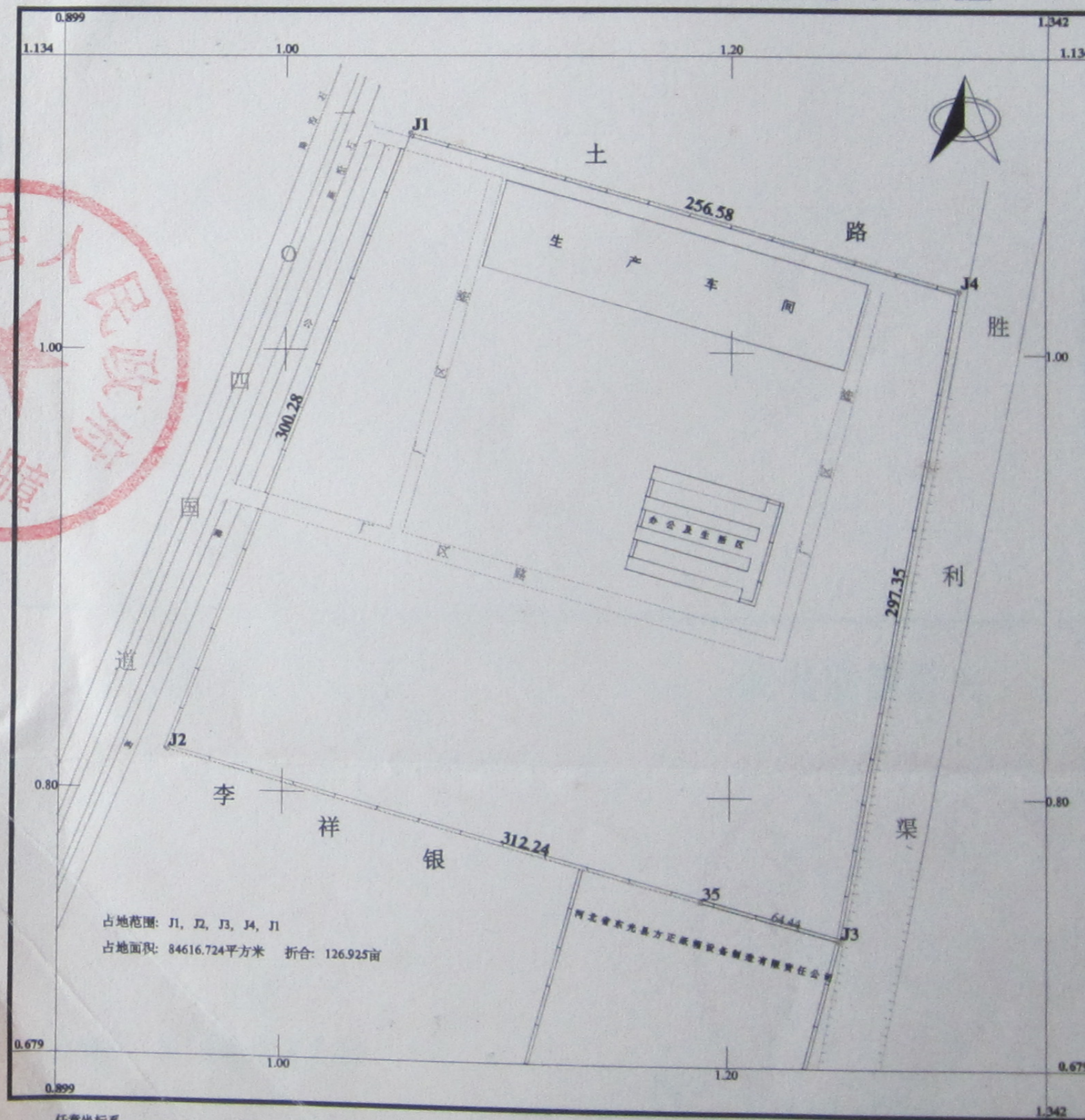
东光县华兴纺织有限责任公司占地平面图
